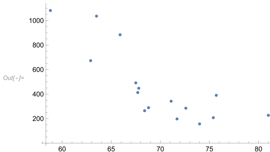
Streudiagramm:
